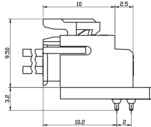
卧式 Right Angle(R-Type)
