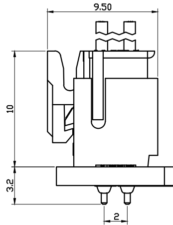
立式 Straight Angle(V-Type)
