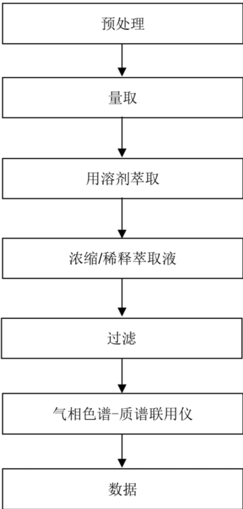
PBBs/PBDEs 检测流程图
