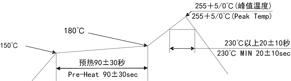
温度条件图
